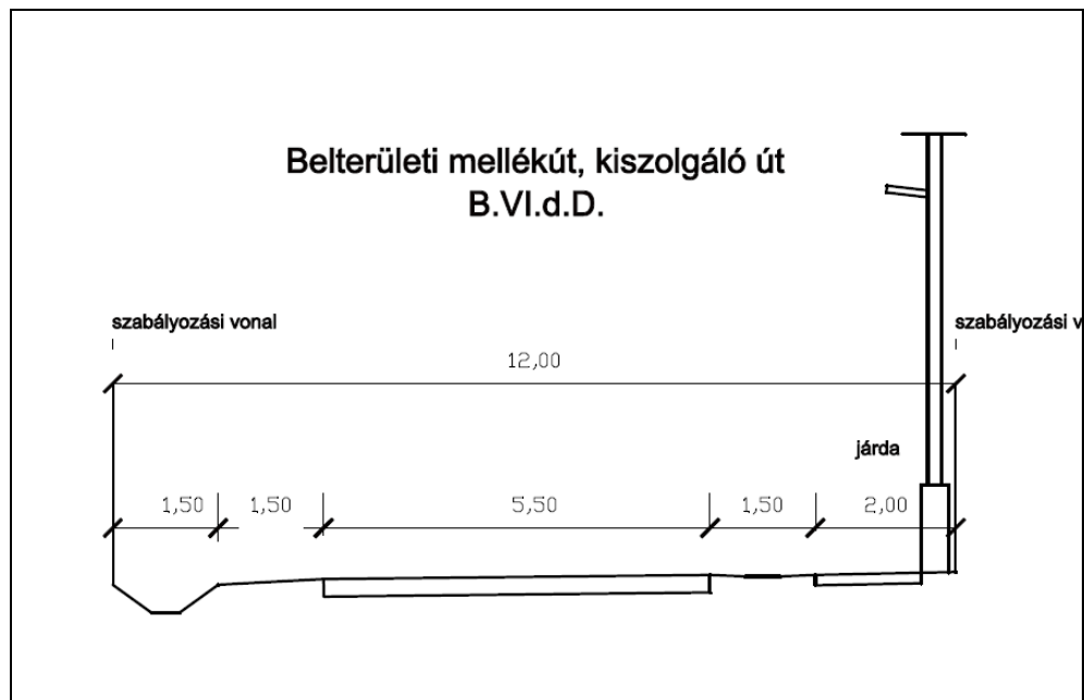
javasolt minta-keresztshelvény
